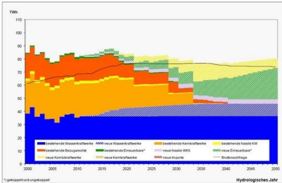
Composizione dell'offerta di elettricità (solo produzione interna) fino al 2020, 2035, 2050 sulla base del presente pacchetto di misure del DATEC (fonte: Prognos)
